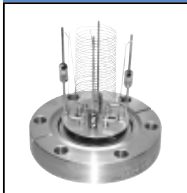
Kratos 84-199R Ion Gauge Filament
